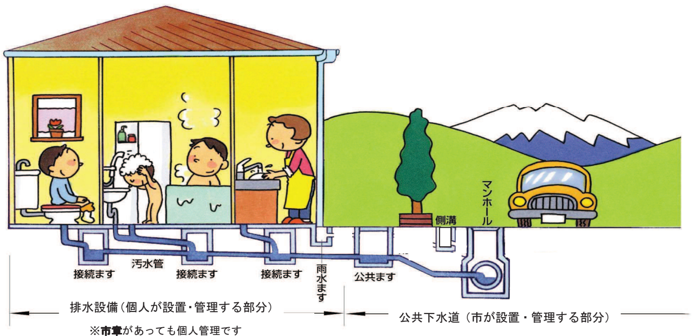
図2：家庭内排水設備の仕組み（分流式）
