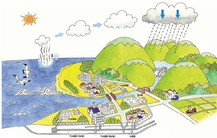
図1：水の循環図
