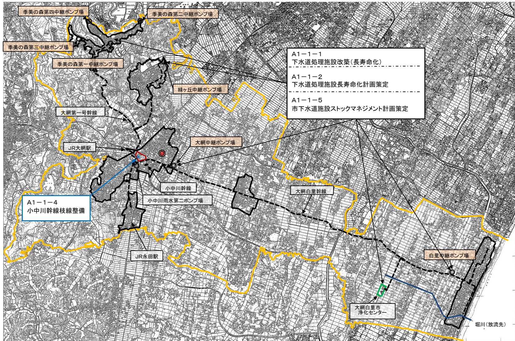
大網白里処理区計画図
